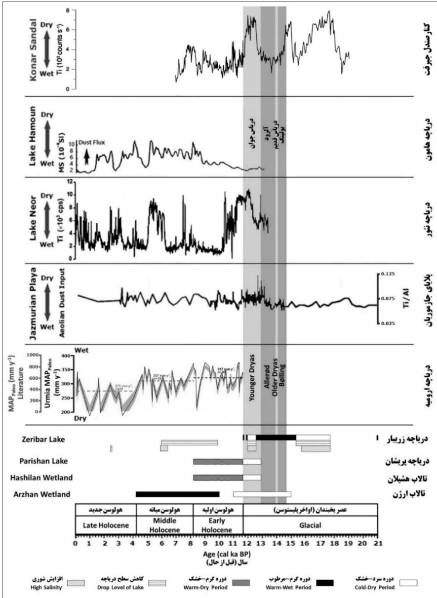
شکل ۳. شرایط اقلیمی اواخر پلیستوسن و هولوسن. محوطه کنارسندل جیرفت، نمودار میزان گردوغبار طی زمان (Safaeirad et al., 2020)؛ دریاچه هامون سیستان، نمودار میزان گردوغبار طی زمان (حمزه و همکاران، ۱۳۹۶)؛ دریاچه نئور اردبیل، نمودار میزان گردوغبار (Sharifi et al., 2015)؛ پلایای جازموریان کرمان، نمودار میزان گردوغبار بادی طی زمان (Vaezi et al., 2019)؛ این نمودارها هر چه به سمت بالا میل کنند، شرایط خشک‌تری را نشان می‌دهند. دریاچه ارومیه در آذربایجان غربی، نمودار میزان بارش سالانه طی زمان که هر چه به سمت بالا میل کند، نشان‌دهنده شرایط اقلیمی مرطوب‌تری است (Sharifi et al., 2019)؛ دریاچه زیربار در استان کردستان (Wasylikova et al., 2006)؛ دریاچه پریشان در استان فارس (داودی و همکاران، ۱۳۹۳)؛ تالاب هشیلان در استان کرمانشاه (صفایی‌راد و همکاران، ۱۳۹۳)؛ تالاب ارزن در استان فارس (سادات حسینی و همکاران، ۱۳۹۵).
